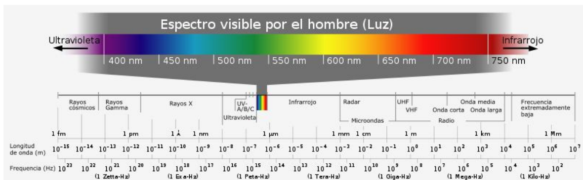
Fig. 1: Espectro electromagnético
