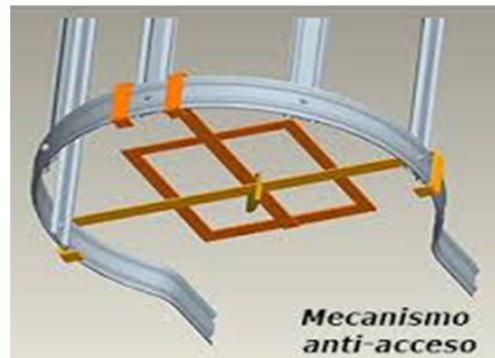
EJEMPLO DE UN MECANISMO DISEÑADO PARA EVITAR ACCESO DE PERSONAL NO AUTORIZADO
